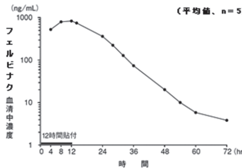
図 フェルビナクパップ70mg 4枚（1枚中にフェルビナク70mgを含有）単回貼付後の血清中フェルビナク濃度推移
