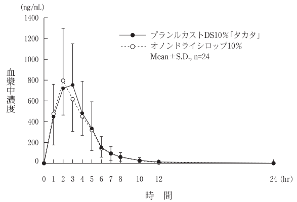
図 16-1 血漿中濃度
